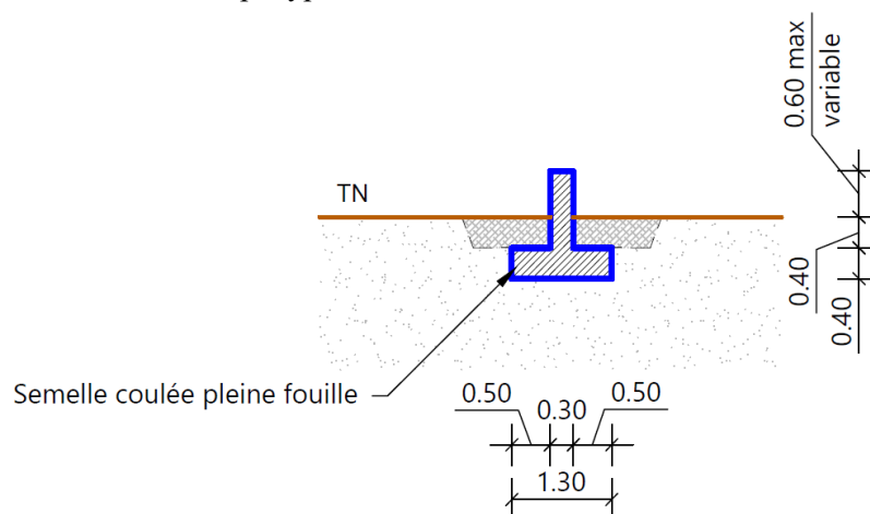
Coupe type du muret – (Source : EGIS/SCP, 2025)
