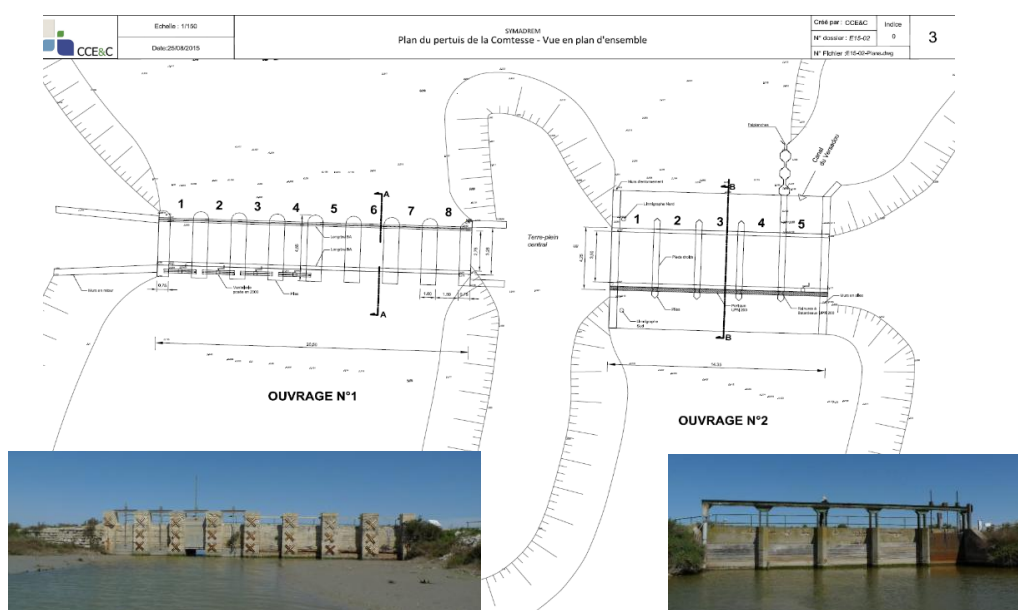
Figure n°2 : Pertuis actuel (vue en plan et photographies)
