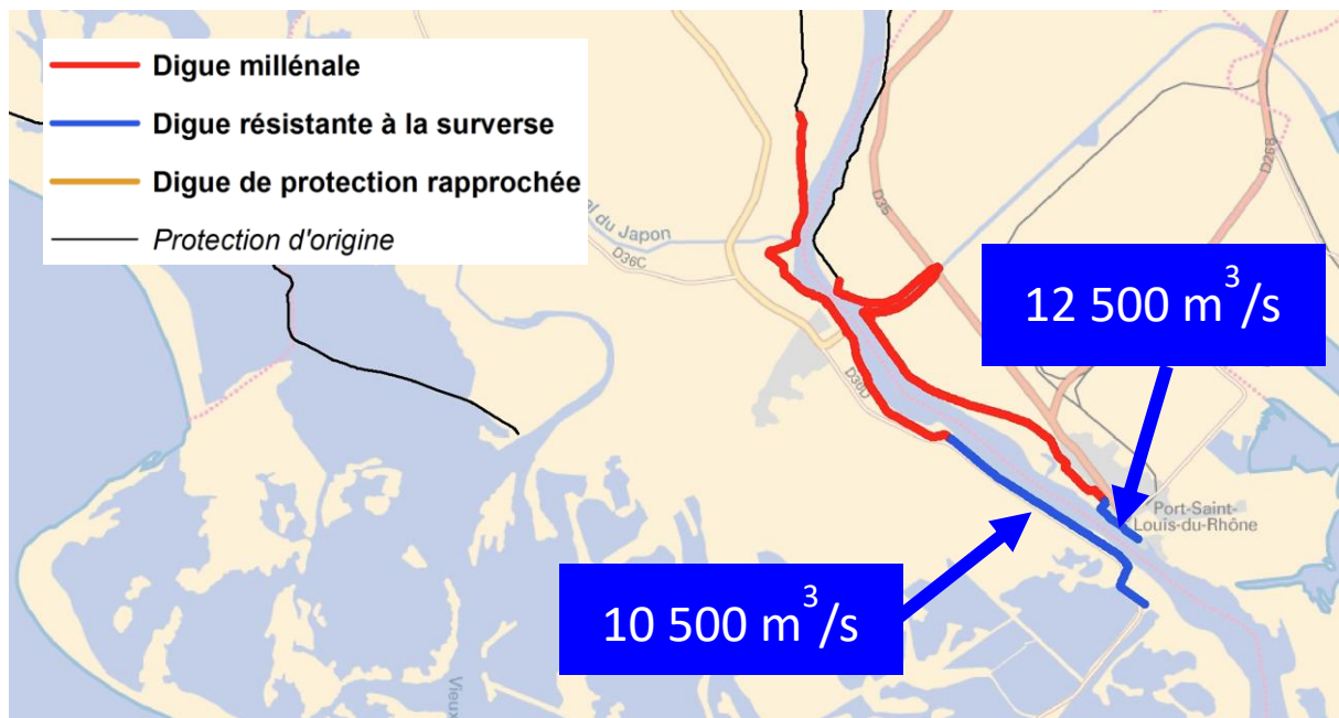
figure n°1 : Principe des travaux
